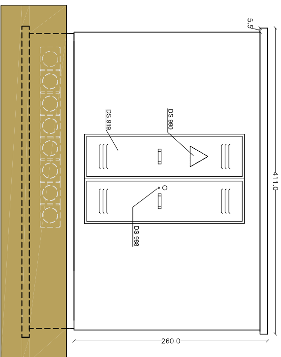
PROSPETTO FRONTALE
