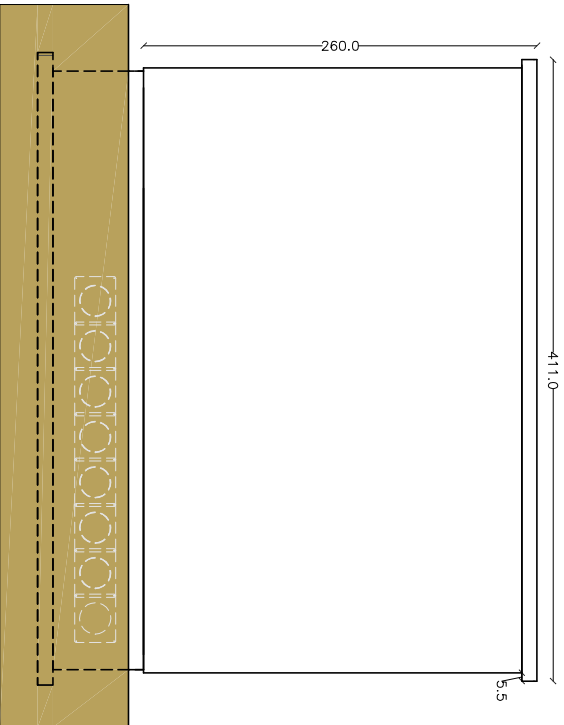
PROSPETTO LATO C
