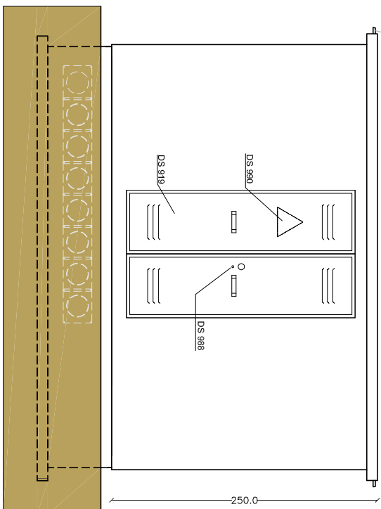
PROSPETTO FRONTALE
