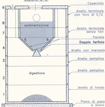
Sezione B-B'
