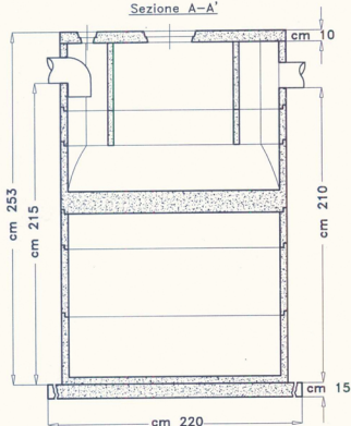
Sezione A-A'
