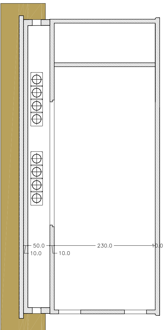
SEZIONE A-A Rapp. 1/50
