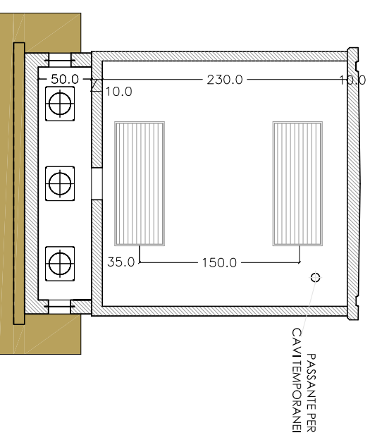
SEZIONE B-B Rapp. 1/20
