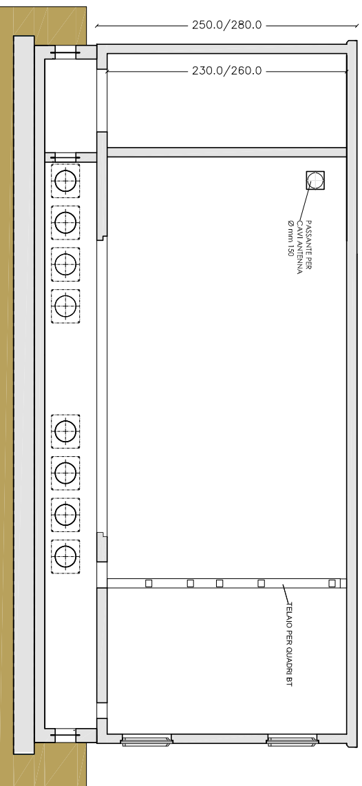
SEZIONE A-A
